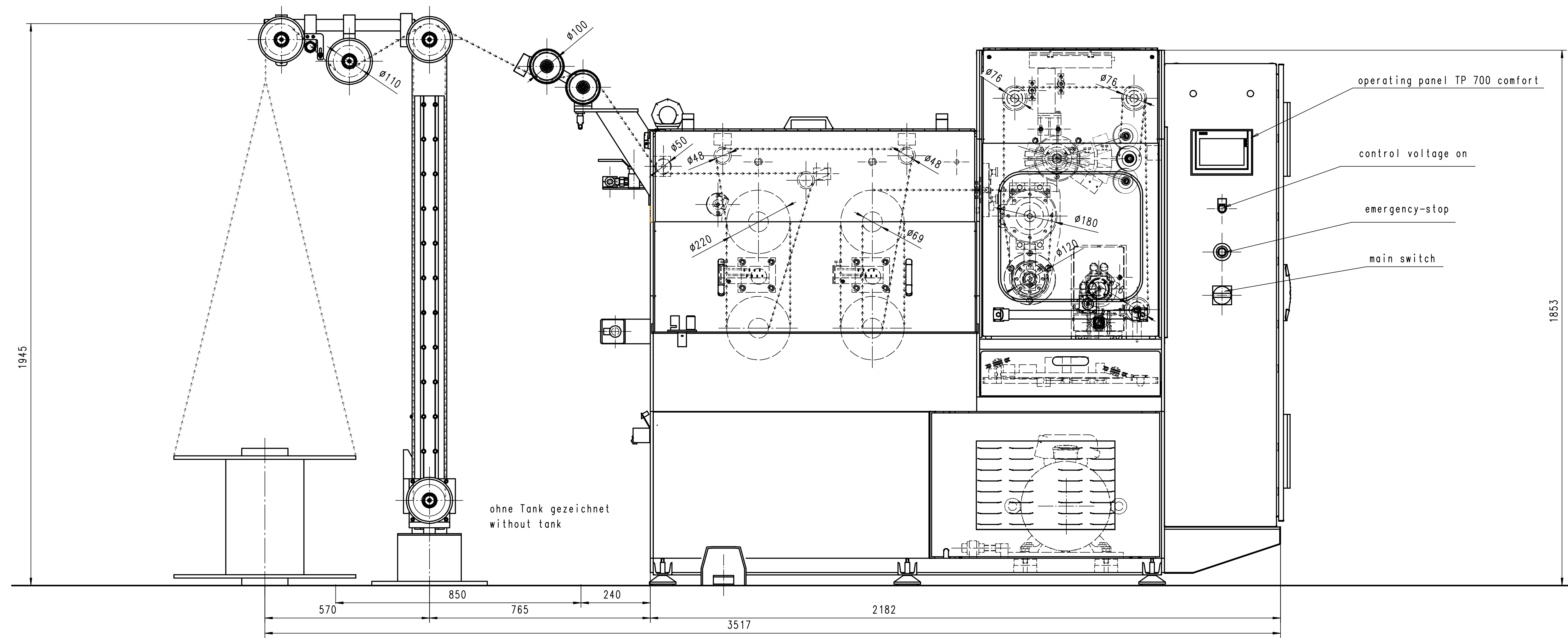
Ablaufständer DAS 1,0/2 Wire pay-off stand DAS 1,0/2
