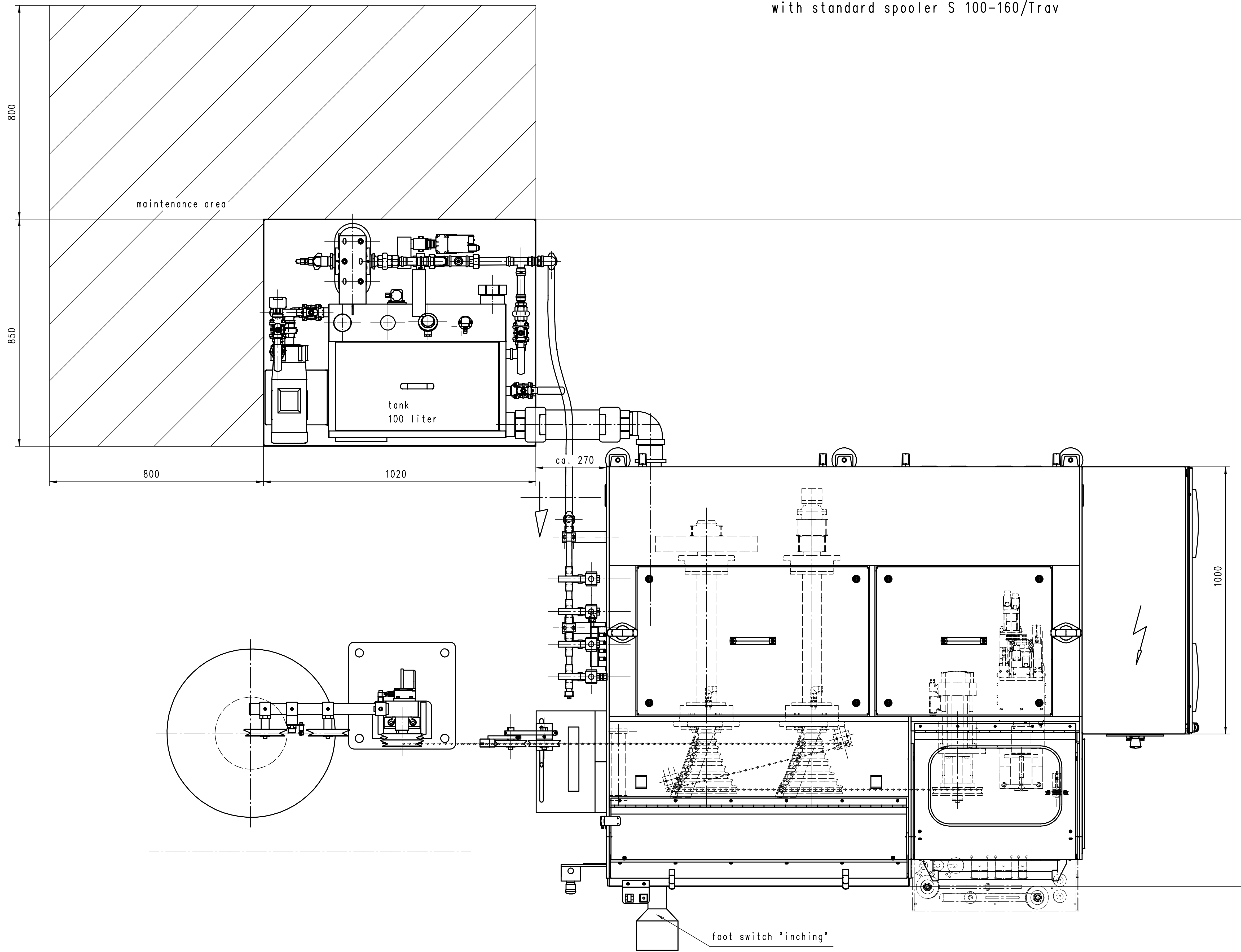
Ablaufständer DAS 1,0/2 Wire pay-off stand DAS 1,0/2
